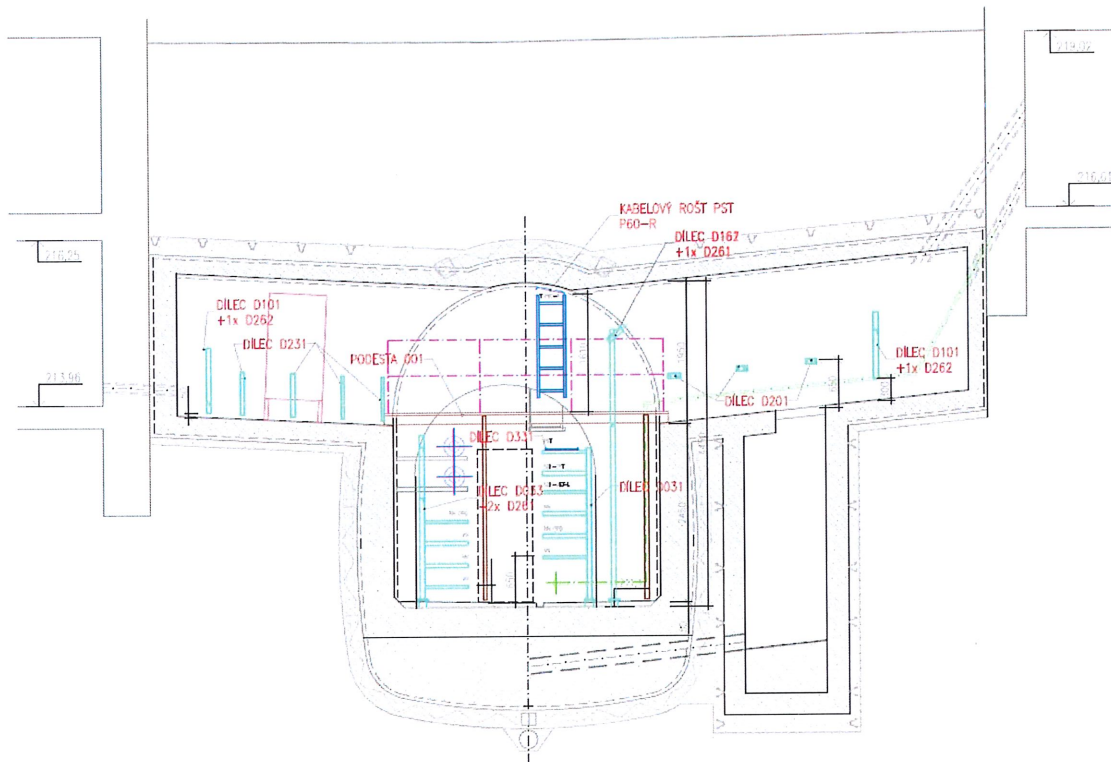
Obr. č. 5 – Příčný řez s vybavením OK a kabelových registrů odbočky Česká 16-18 a Česká 19
