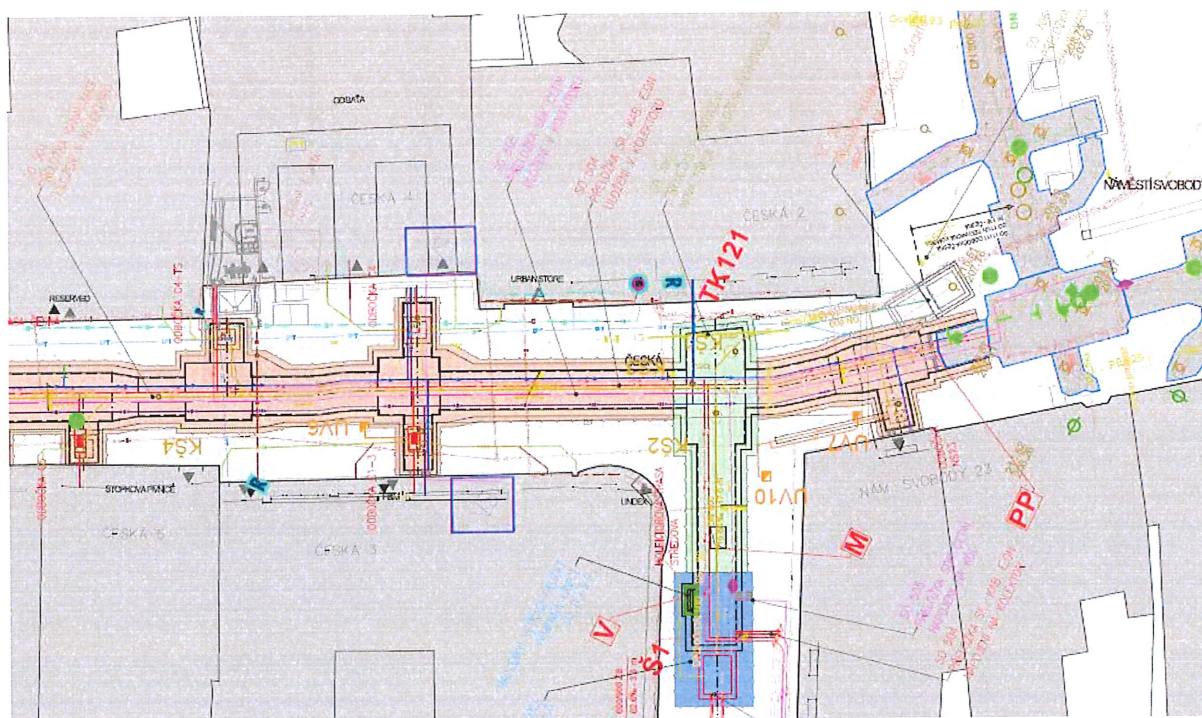
Obr. č. 1 – Část situace stavby – napojení na stávající kolektor nám. Svobody – Česká – Středova
